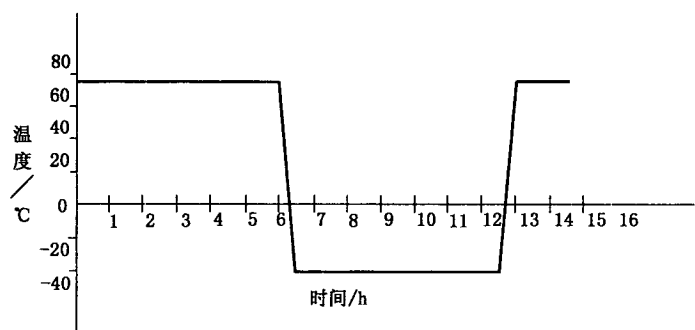
图 1 温度循环流程示意图
